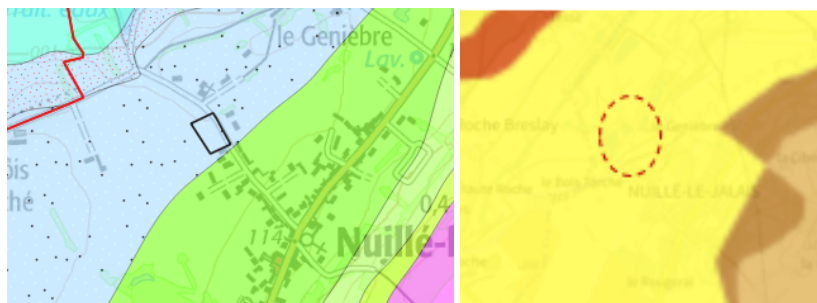
Figure 5 : Extraits de la carte géologique de France (source : infoterre) et de la carte des sols de France (source : Géoportail)
